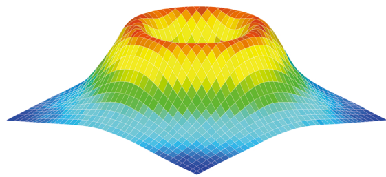
인체에 발생하는 유도 전기장
