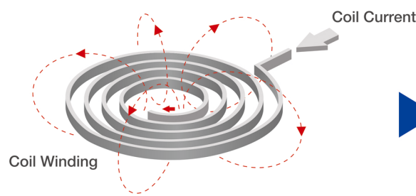
Coil wire에서 발생하는 유도 자기장
